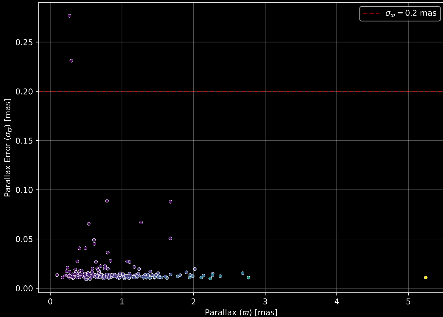
GALAH DR4 Field: [8389] Parallax Quality (n= 246)
