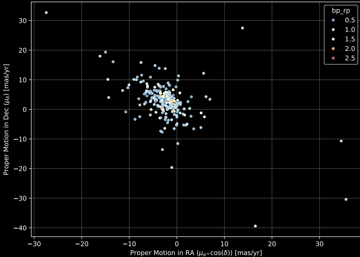
GALAH DR4 Field: [8389] Proper Motion Diagram (n= 246)
