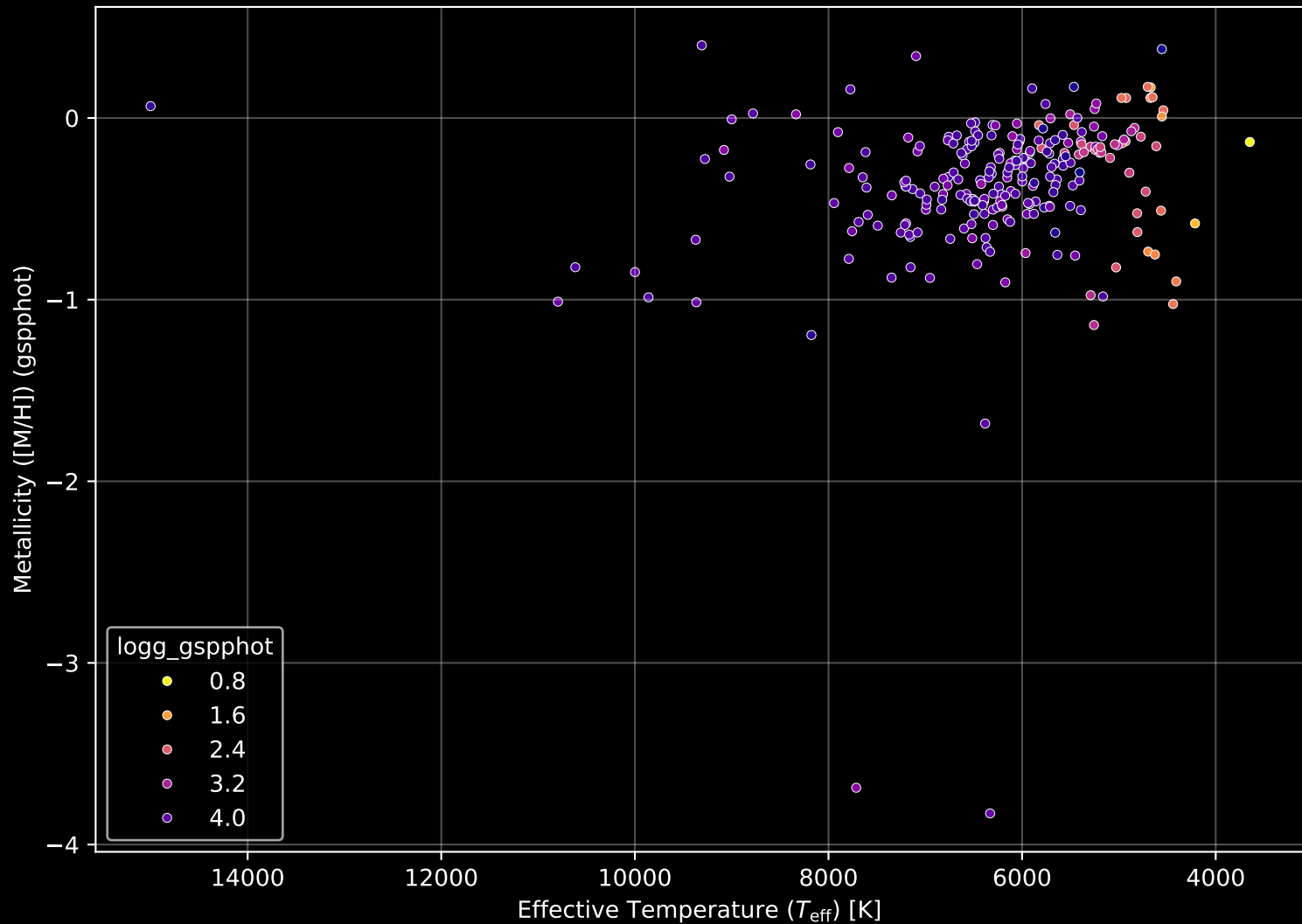
GALAH DR4 Field: [8389] Stellar Population Parameters (n= 246)
