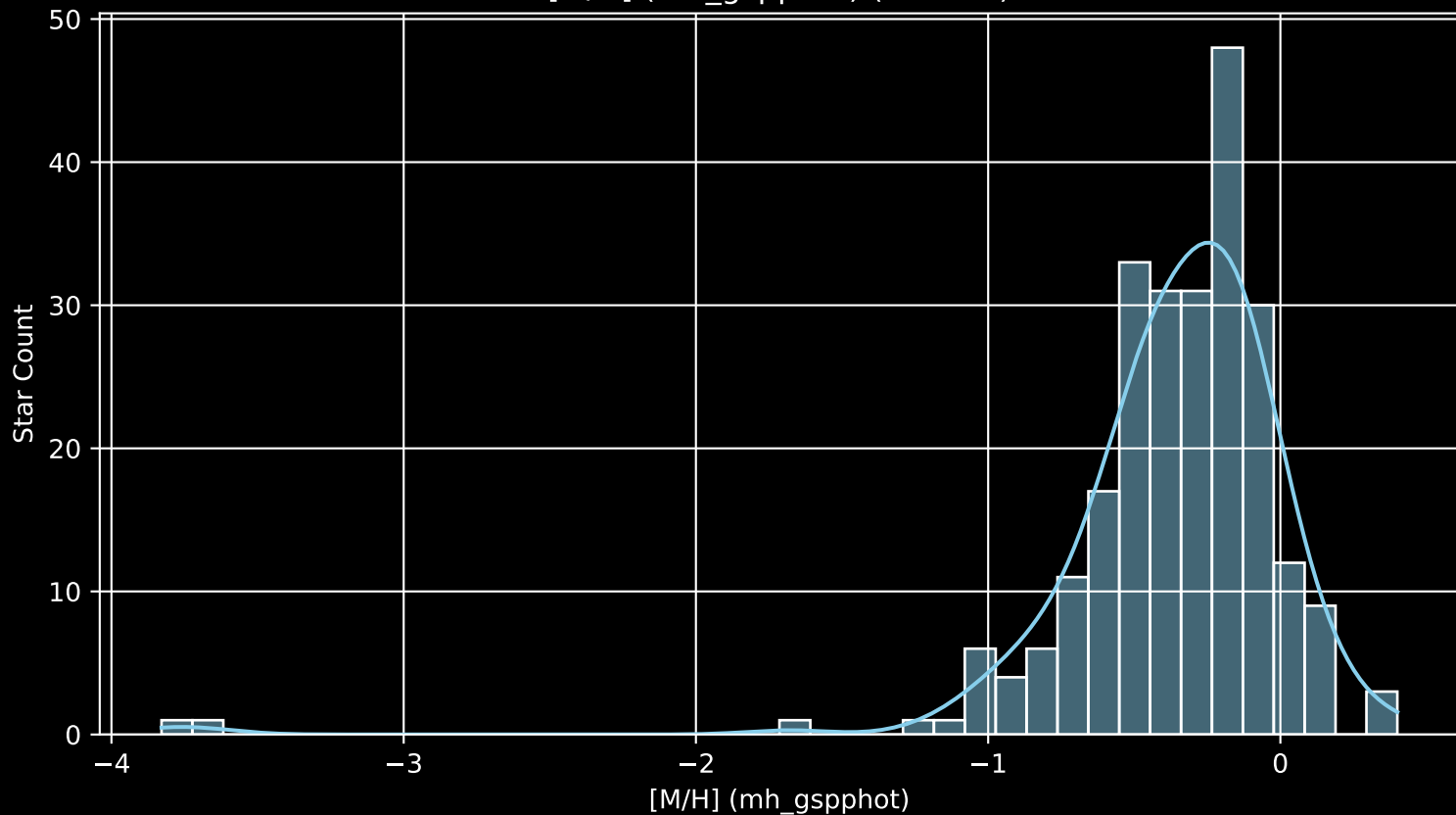
GALAH DR4 Field: [8389] [M/H] (mh_gspphot) (n= 246)
