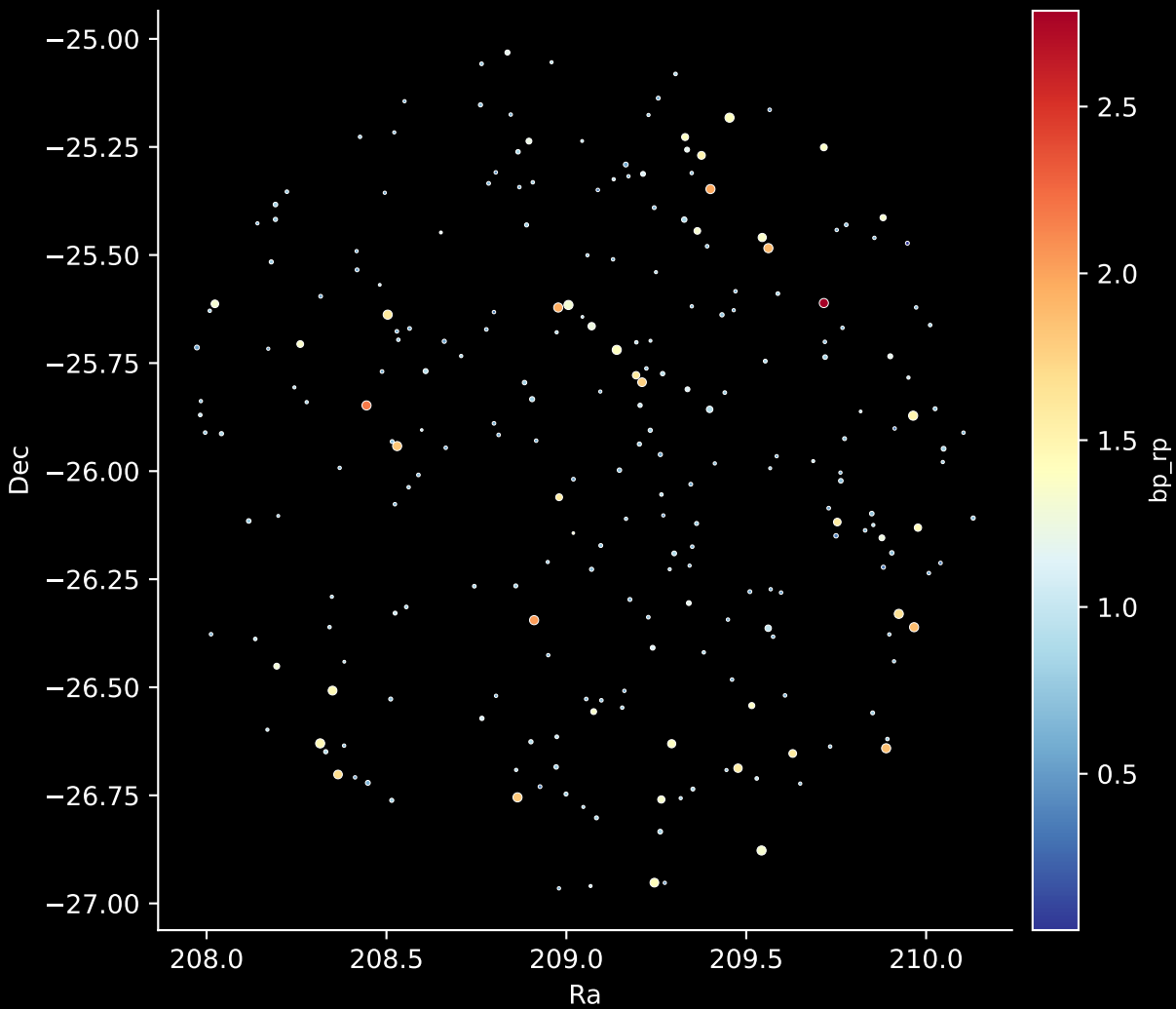
GALAH DR4 Field: [8389] Stars: 246
